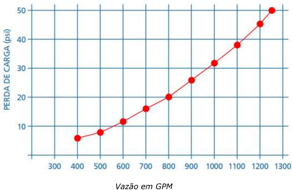
Gráfico de perda de carga
